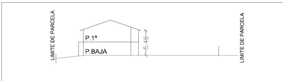
SECCION B-B
